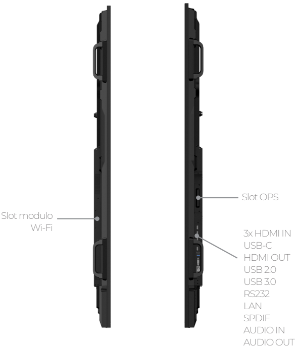
Pannelli laterali
