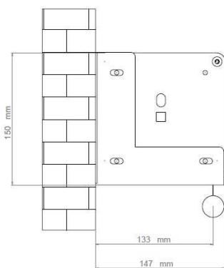
Fissaggio a parete con caduta tela anteriore
