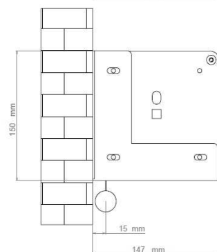
Fissaggio a parete con caduta tela posteriore
