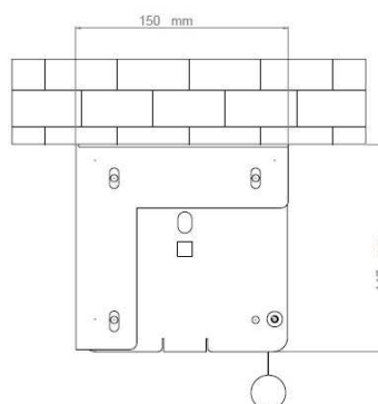
Fissaggio a soffitto
