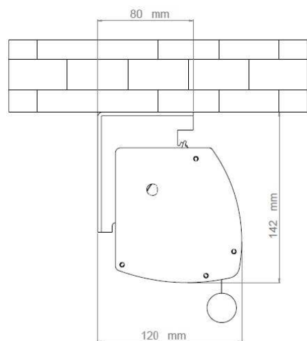
Fissaggio a soffitto
