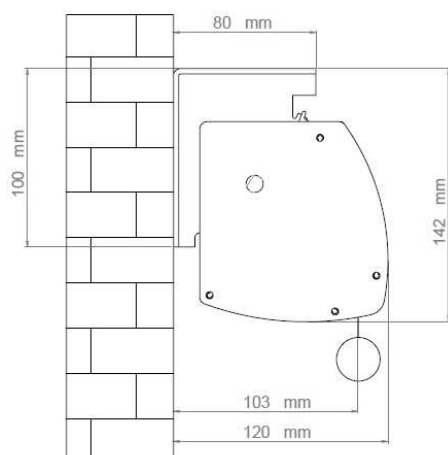
Fissaggio a parete
