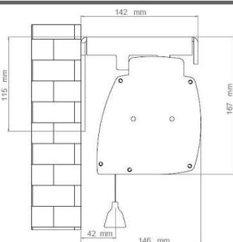
Installazione a parete - caduta tela posteriore
