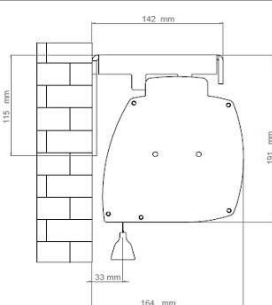
Installazione a parete - caduta tela posteriore
