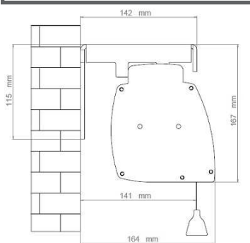
Installazione a parete - caduta tela frontale
