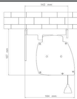
Installazione a soffitto
