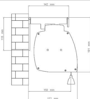
Installazione a parete - caduta tela frontale
