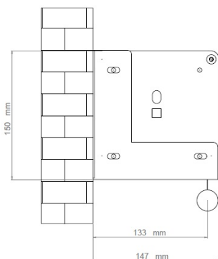
Fissaggio a parete con caduta tela anteriore
